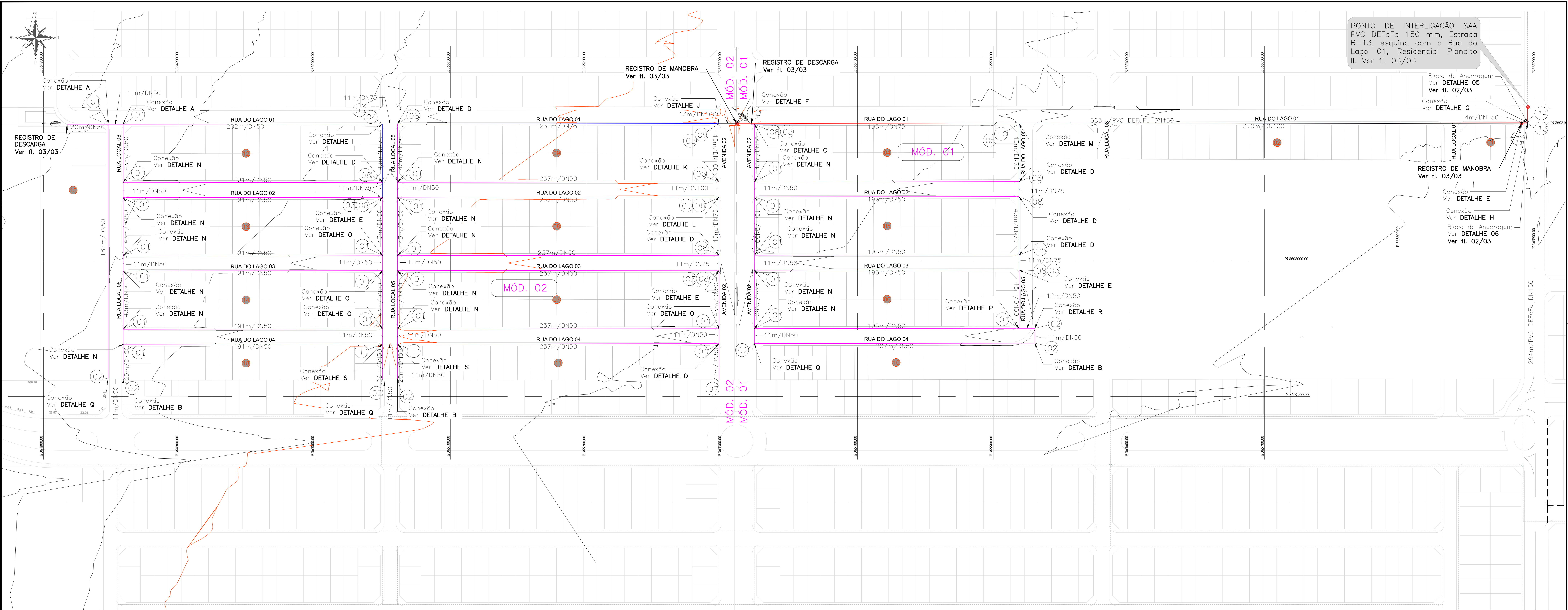
PLANTA BAIXA - REDE DE DISTRIBUIÇÃO PRINCIPAL E SECUNDÁRIA ESC. 1:1000
