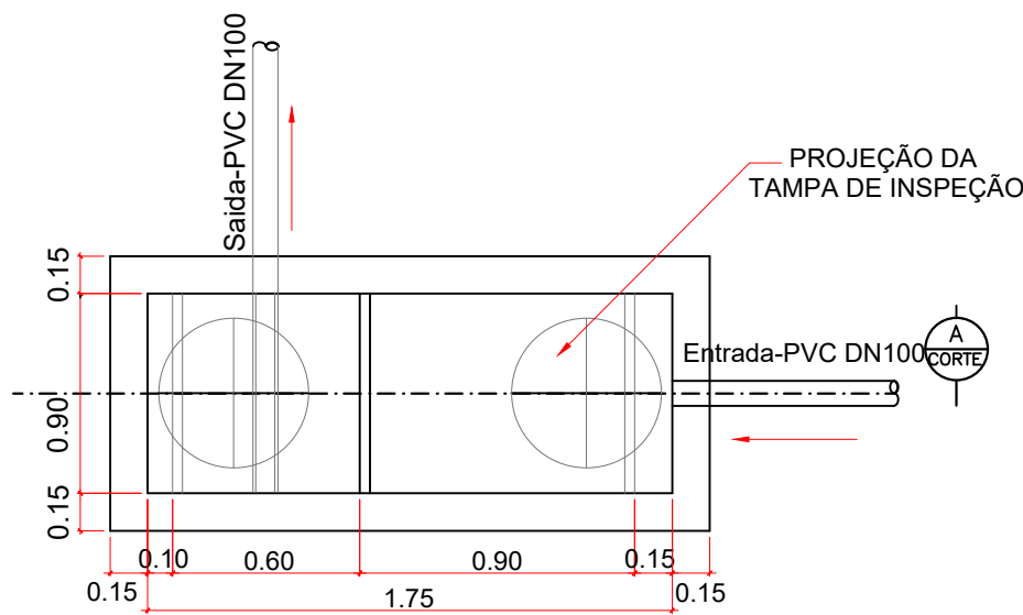
01 FOSSA SÉPTICA SEM ESCALA
