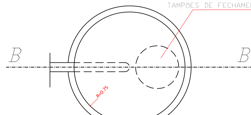
04 PLANTA SUMIDOURO SEM ESCALA
