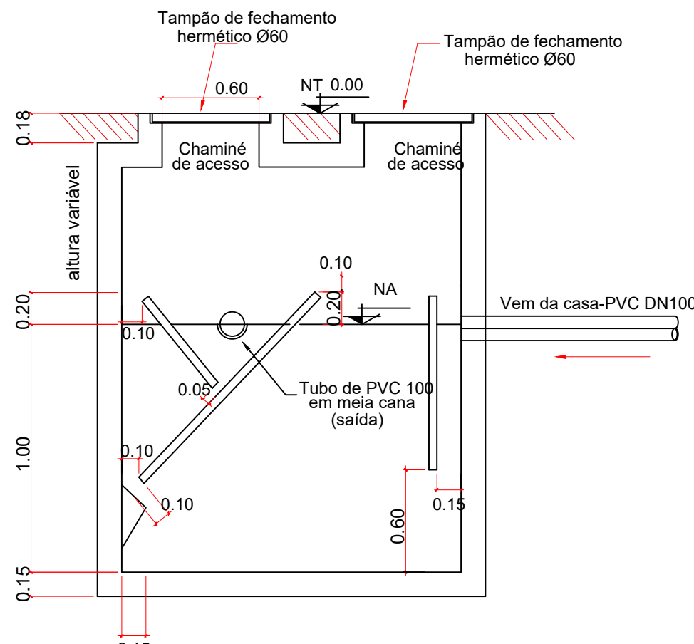
03 CORTE AA SEM ESCALA
