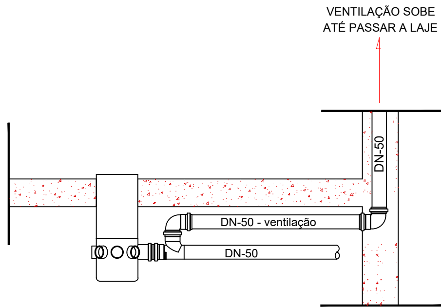
02 DETALHE TUBO DE VENTILAÇÃO SEM ESCALA
