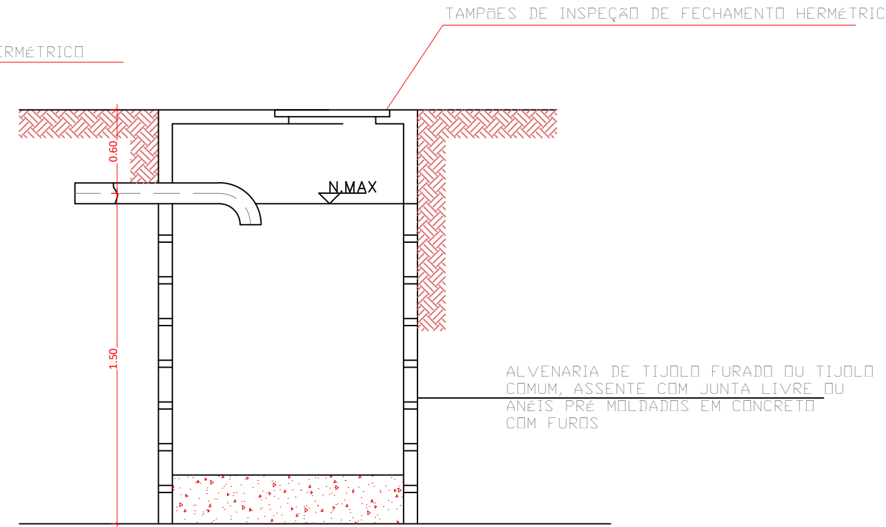
05 CORTE BB SEM ESCALA
