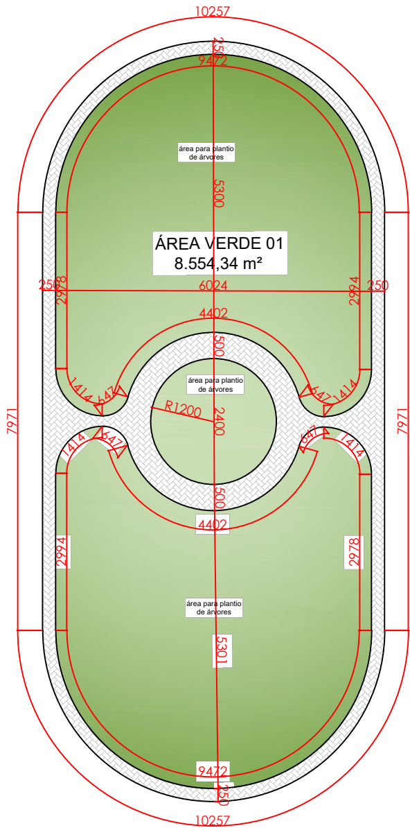
02 PLANTA BAIXA SETORIZAÇÃO ESC: 1/1000
