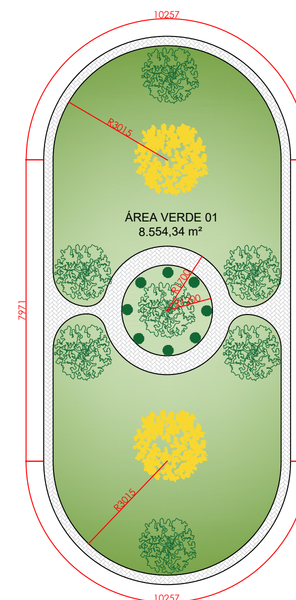
03 PLANTA BAIXA PLANTIO ESC: 1/1000
