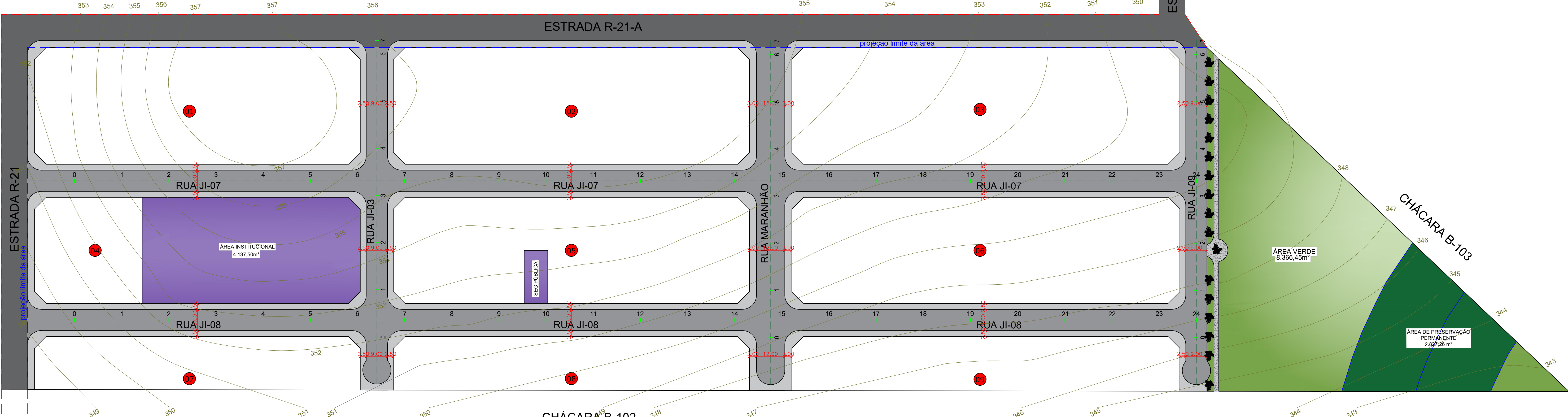
PLANTA DE PAVIMENTAÇÃO 1 : 1000
