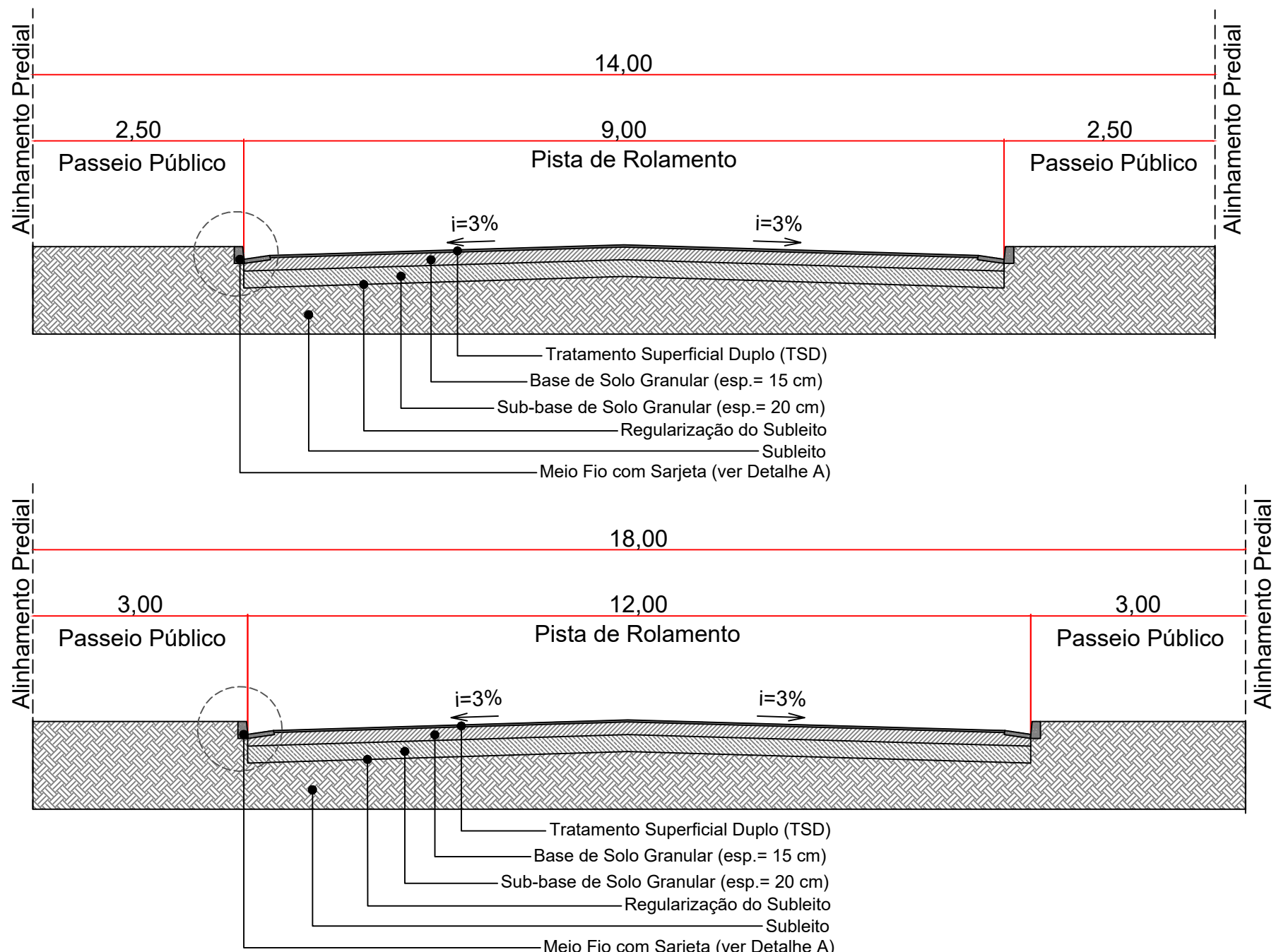
DETALHES SEÇÃO SEM ESCALA
