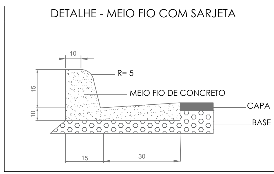
DETALHE - MEIO-FIO SEM ESCALA
