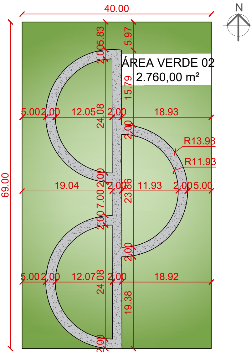
PLANTA BAIXA ÁREA VERDE 02 - DIMENSÕES 1 : 500
