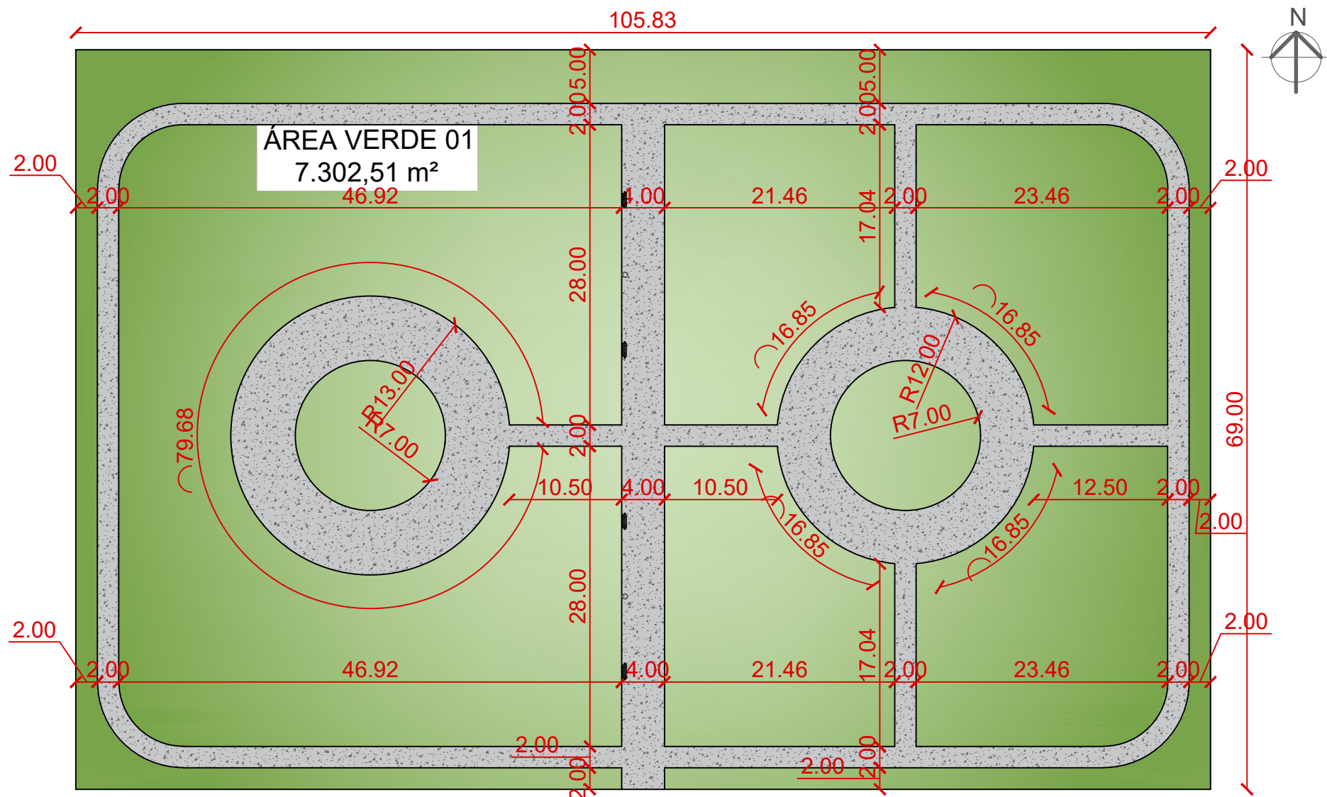
PLANTA BAIXA ÁREA VERDE 01 - DIMENSÕES 1 : 500
