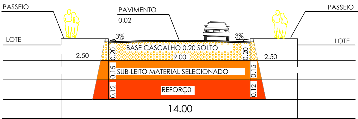
SECÇÃO TRANSVERSAL DAS RUAS DE 9.00m
