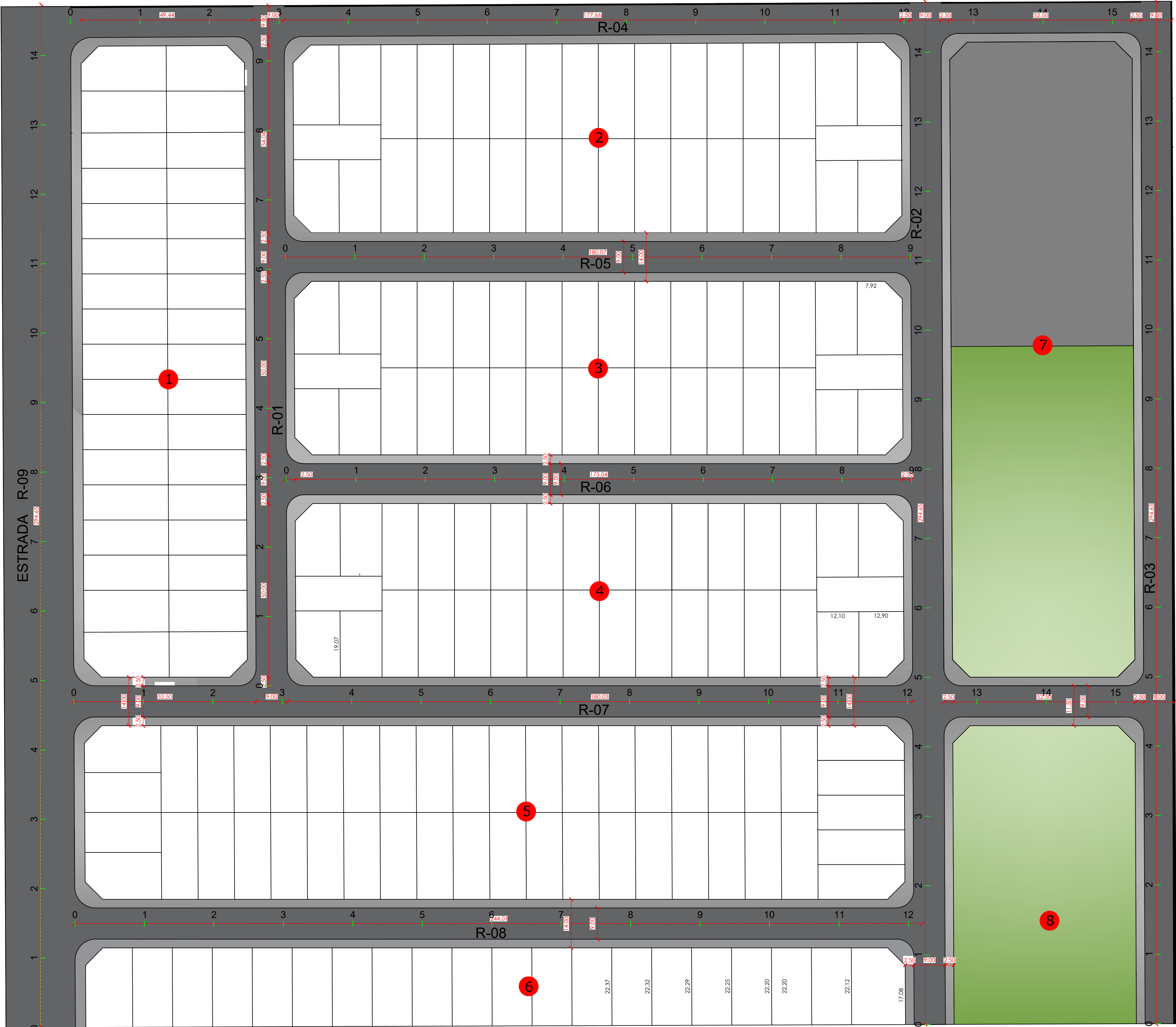
1 PLANTA BAIXA PAVIMENTAÇÃO ESC: 1/700
