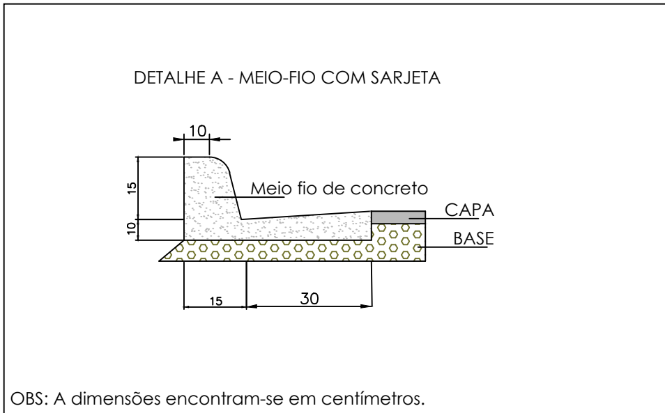
3 DETALHE MEIO FIO SEM ESCALA
