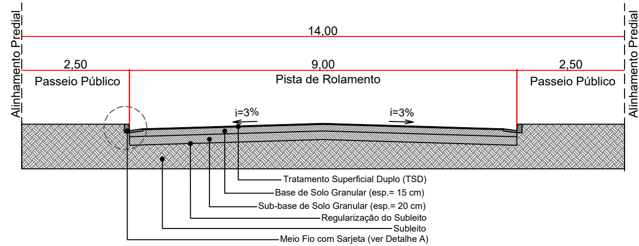
2 DETALHE SEÇÃO SEM ESCALA
