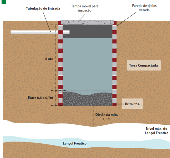
Figura 3 – Sumidouro Circular
