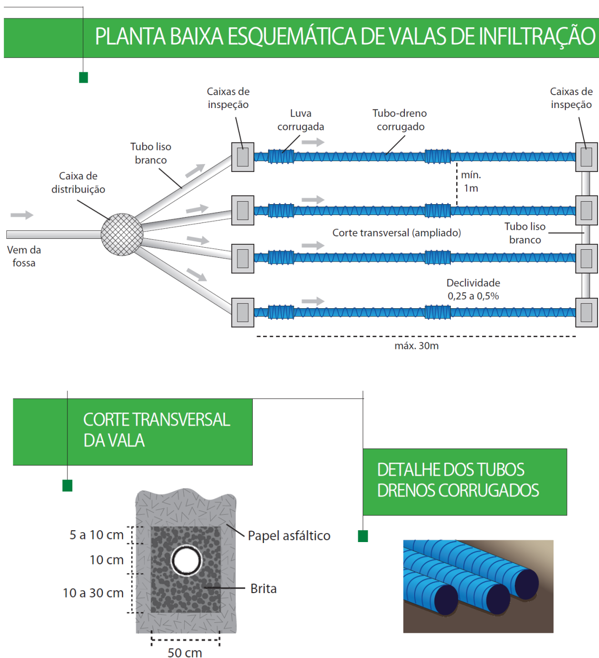
Figura 4 – Valas de Infiltração
