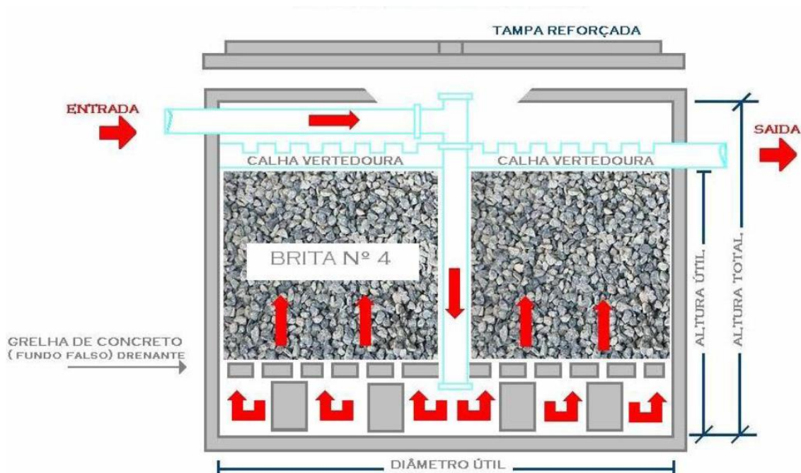
Figura 6 – Filtro anaeróbio com fundo falso
