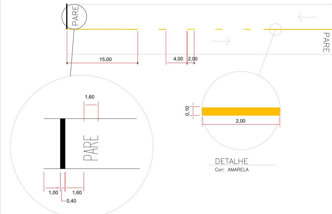
DETALHE DA SINALIZAÇÃO HORIZONTAL
