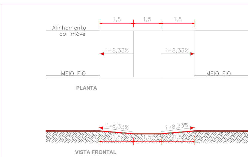
REBAIXAMENTO DE CALÇADAS ESTREITAS
