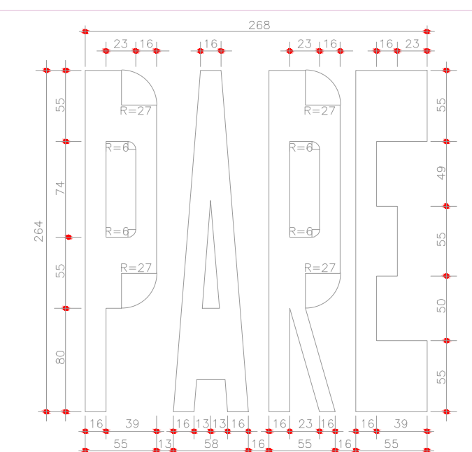
DIAGRAMAÇÃO DA LEGENDA "PARE"
