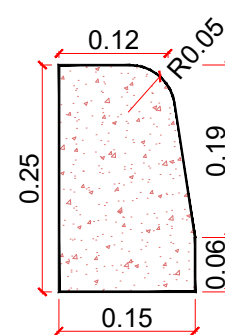
DETALHE DO MEIO-FIO S/E
