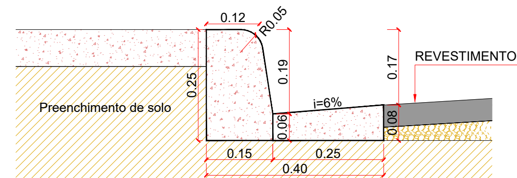
DETALHE DA SARJETA E MEIO-FIO S/E
