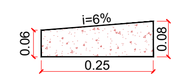
DETALHE DA SARJETA S/E
