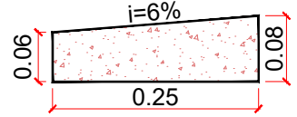
DETALHE DA SARJETA S/E
