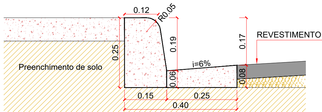
DETALHE DA SARJETA E MEIO-FIO S/E
