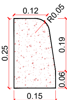
DETALHE DO MEIO-FIO S/E
