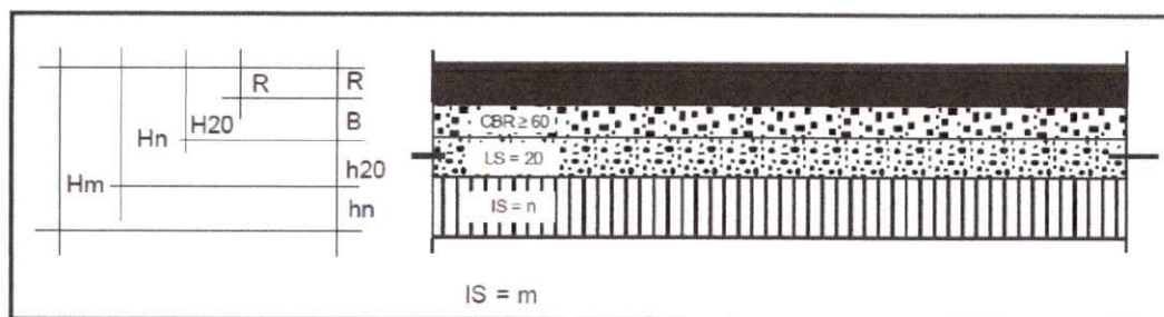
Estrutura da seção total do pavimento
