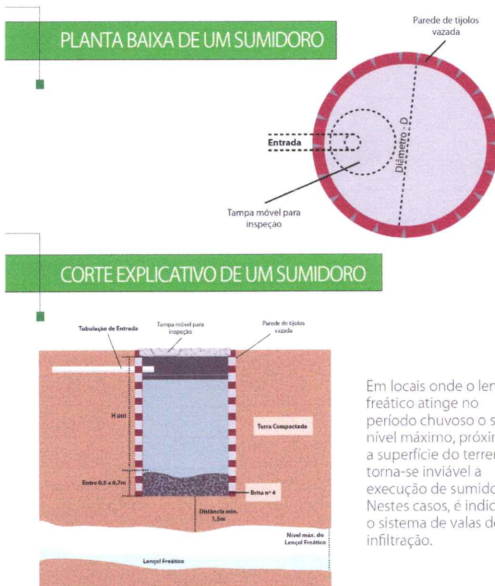
Figura 3 – Sumidouro Circular
