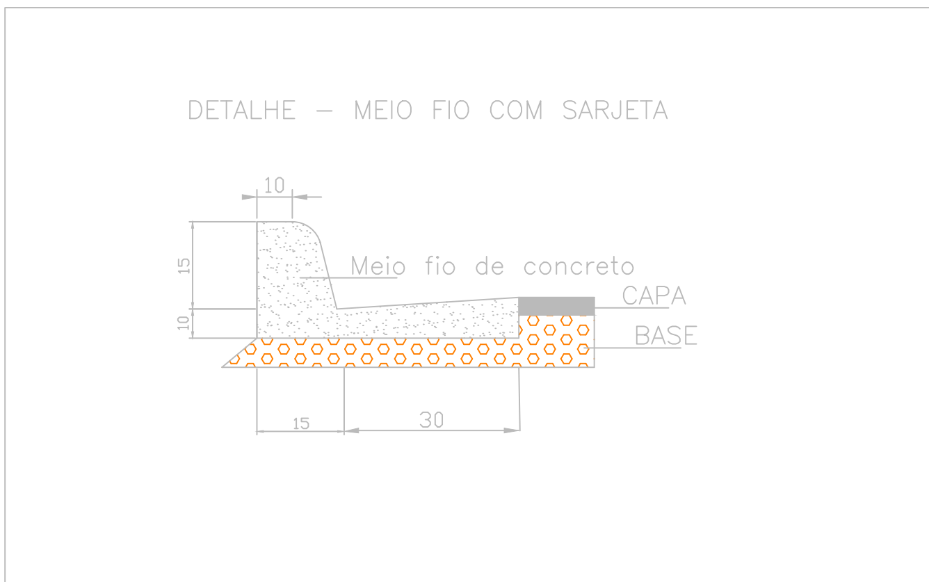
2 Detalhe - Meio-Fio Sem Escala
